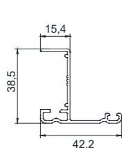
Profil du battant
