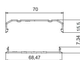
Profil base écharpes
