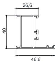
Profil Précadre
