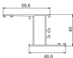
Profil Précadre avec recouvrement
